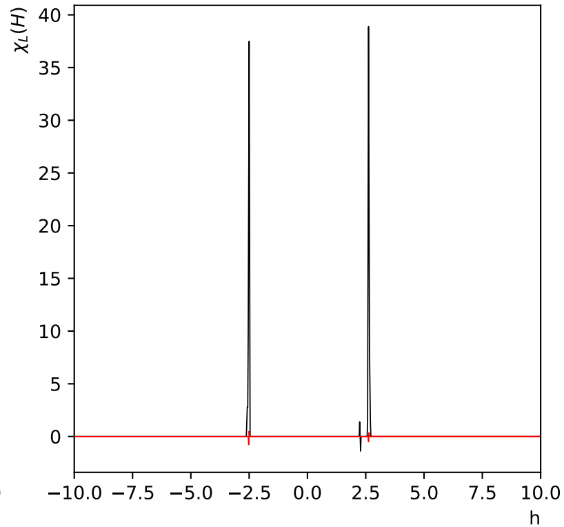
\chi_L(H) réseau de taille L=6 à T=0.5
