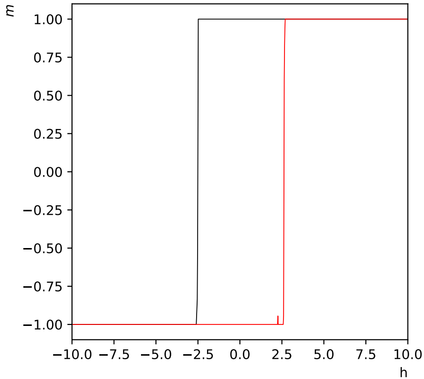
Hystérésis de l'aimantation réseau de taille L=6 - h=10 à T=0.5
